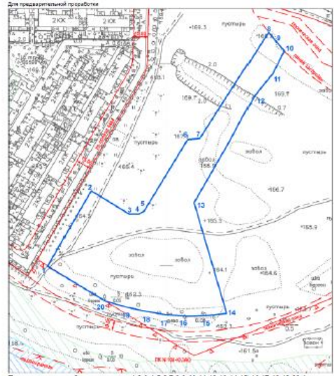
СИТУАЦИОННЫЙ ПЛАН 1:2000
